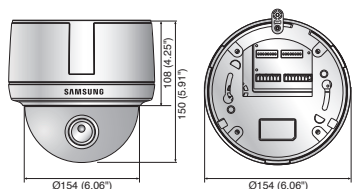
SCP-3120
