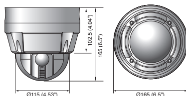
SCP-3120V
